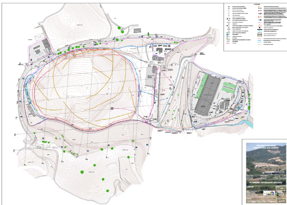
Figura 4 Rete drenante
