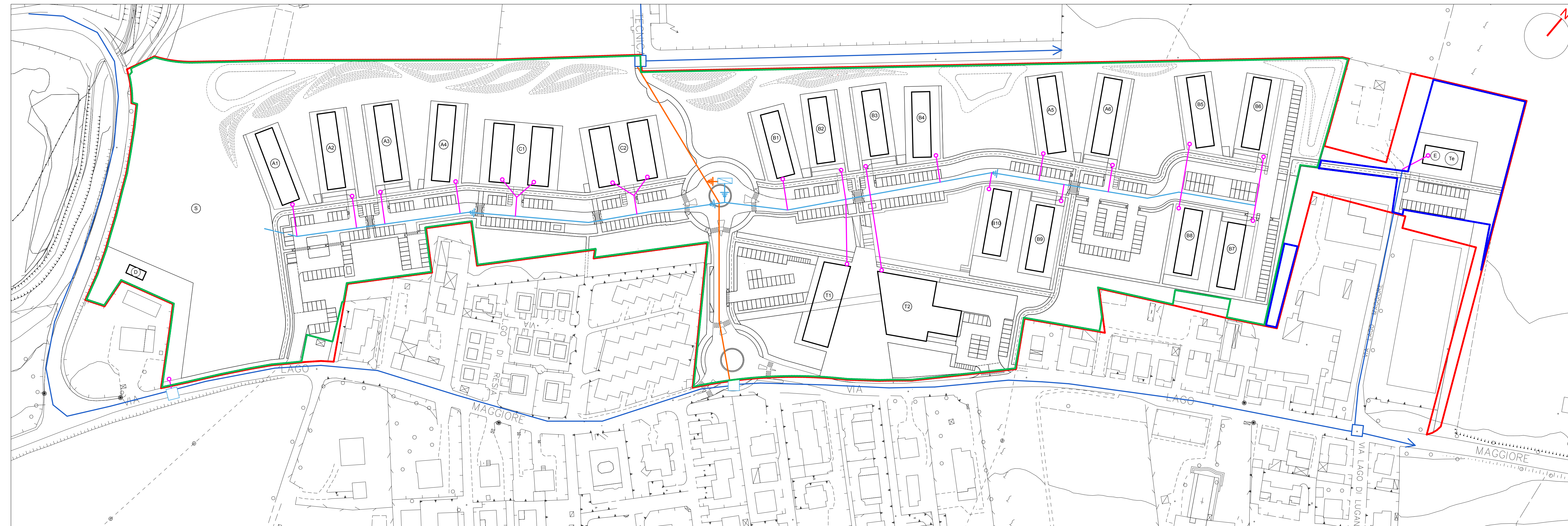
URBANIZZAZIONE RETE GAS SCALA 1:1000
