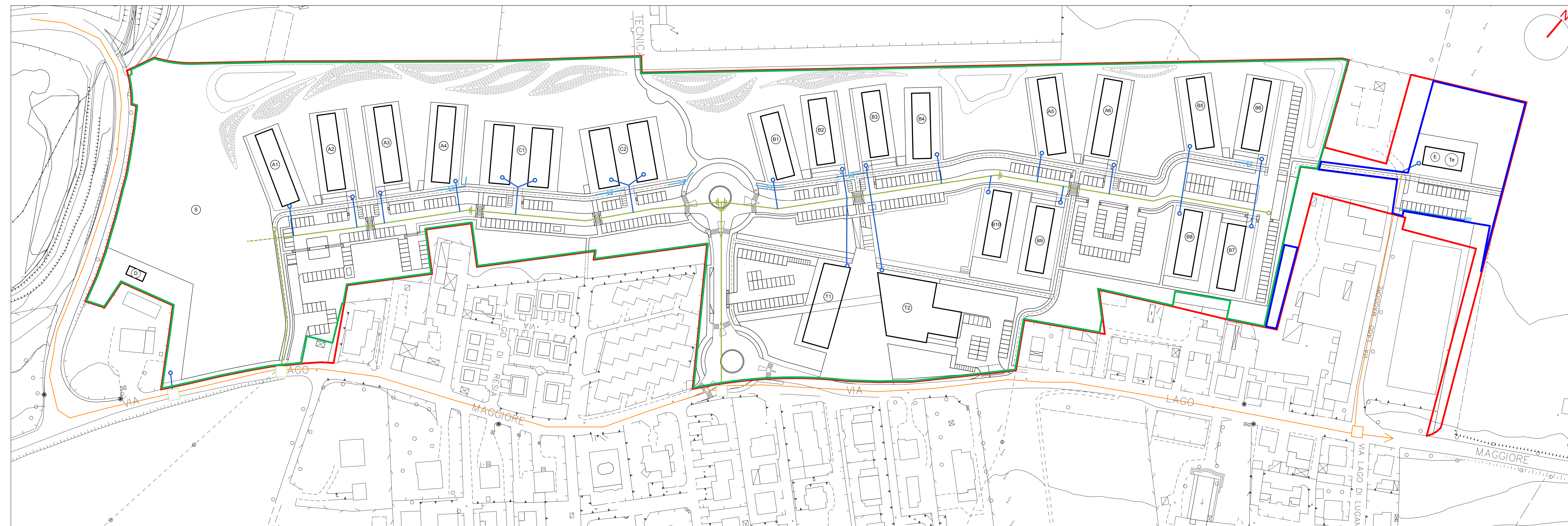
URBANIZZAZIONE RETE IDRICA SCALA 1:1000
