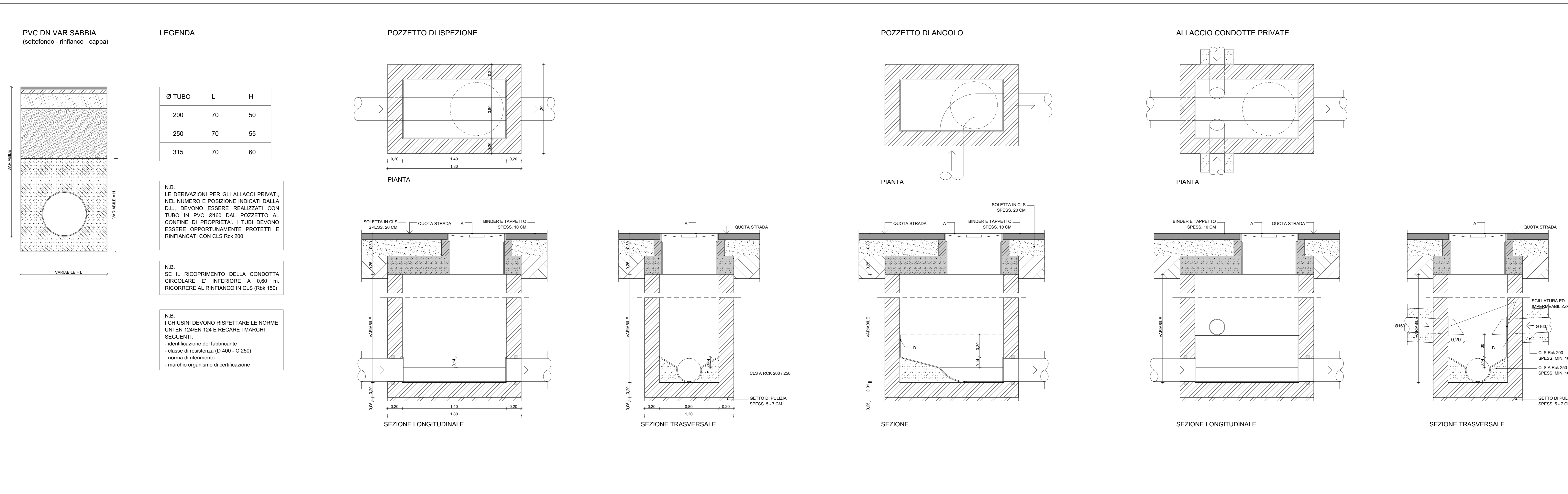
PARTICOLARI FOGNATURA NERA, ALLACCI SCALA 1:20
