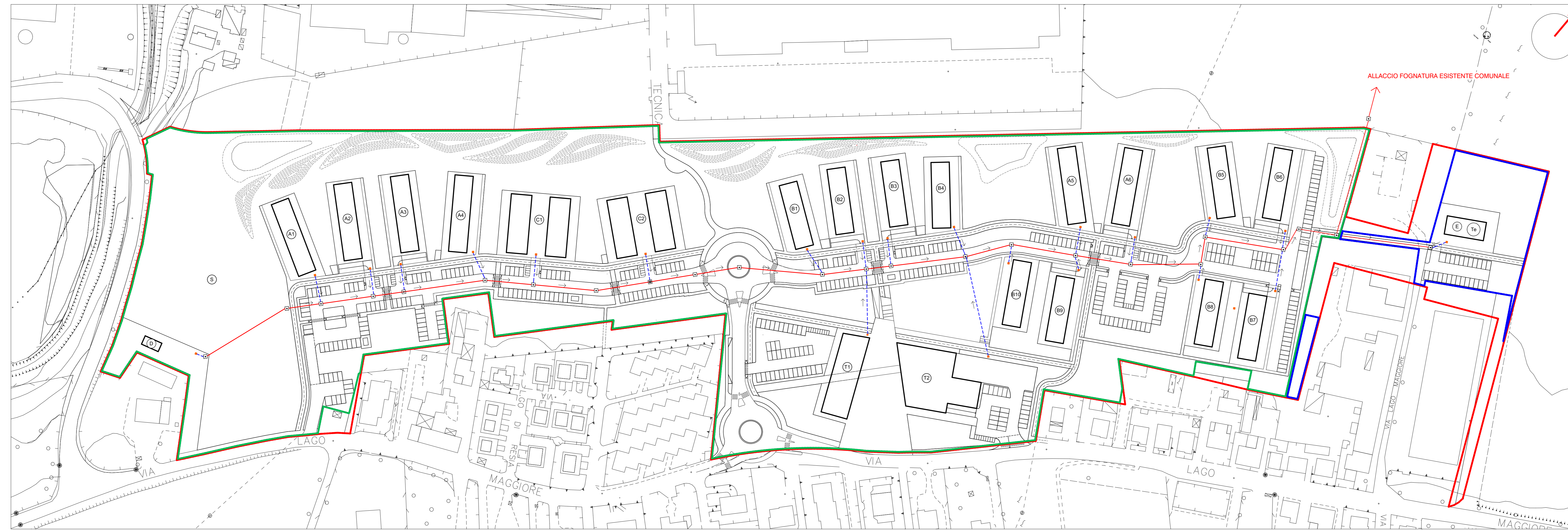
URBANIZZAZIONE FOGNATURA NERA, PLANIMETRIA SCALA 1:1000
