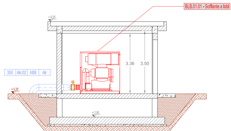
SEZIONE B-B
