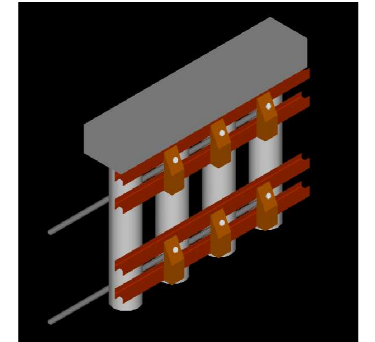
PARTICOLARE PROSPETTO PARATIA TIRANTATA
