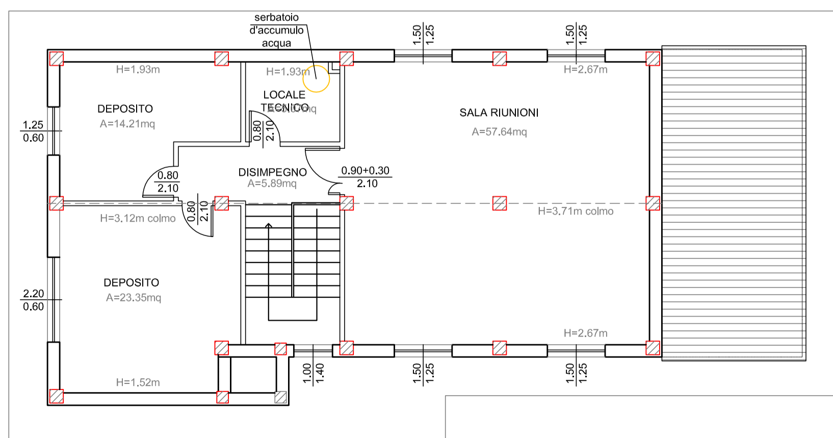
PLANIMETRIA PIANO PRIMO scala 1:100
