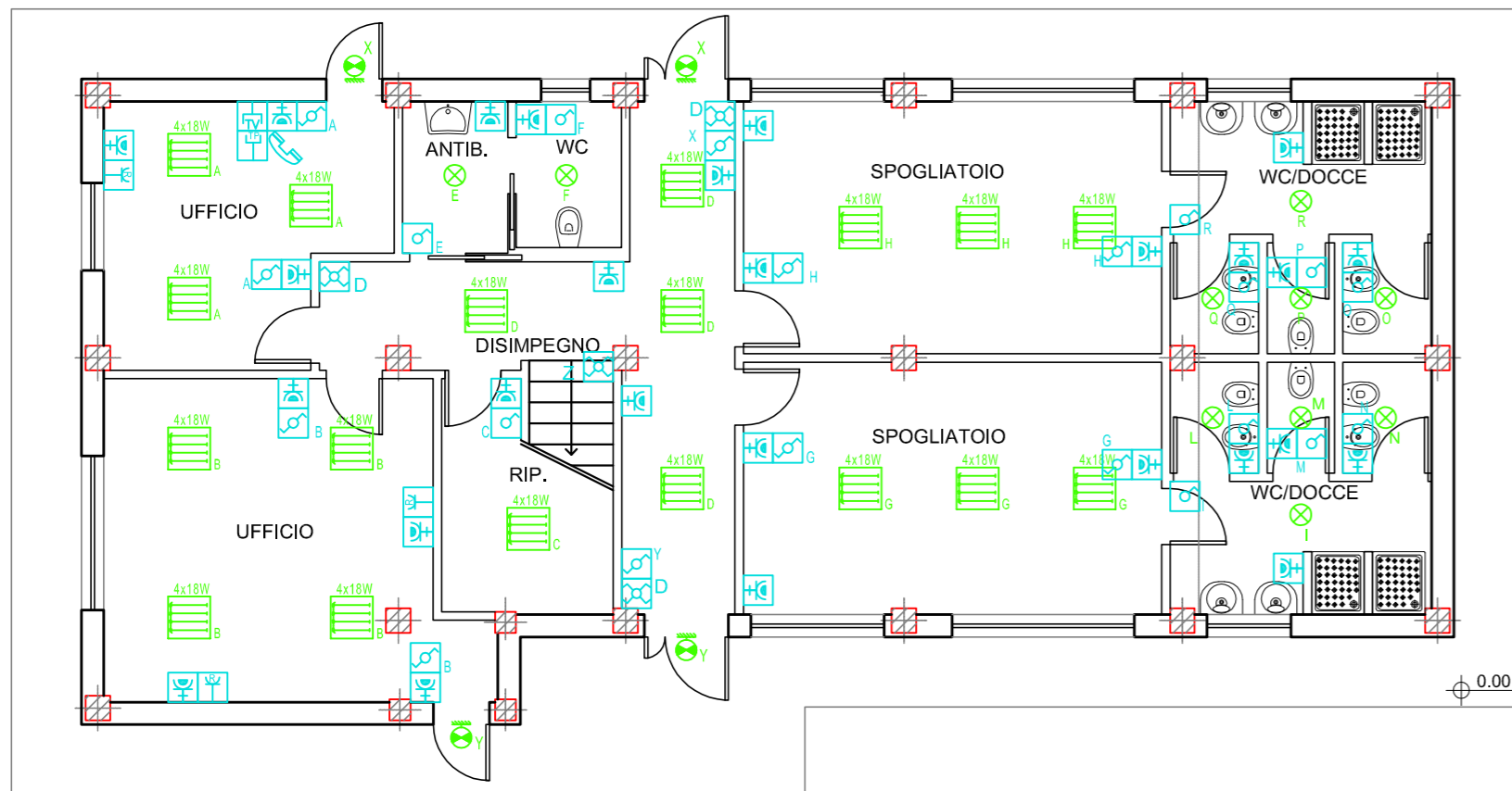
PLANIMETRIA PIANO TERRA scala 1:100
