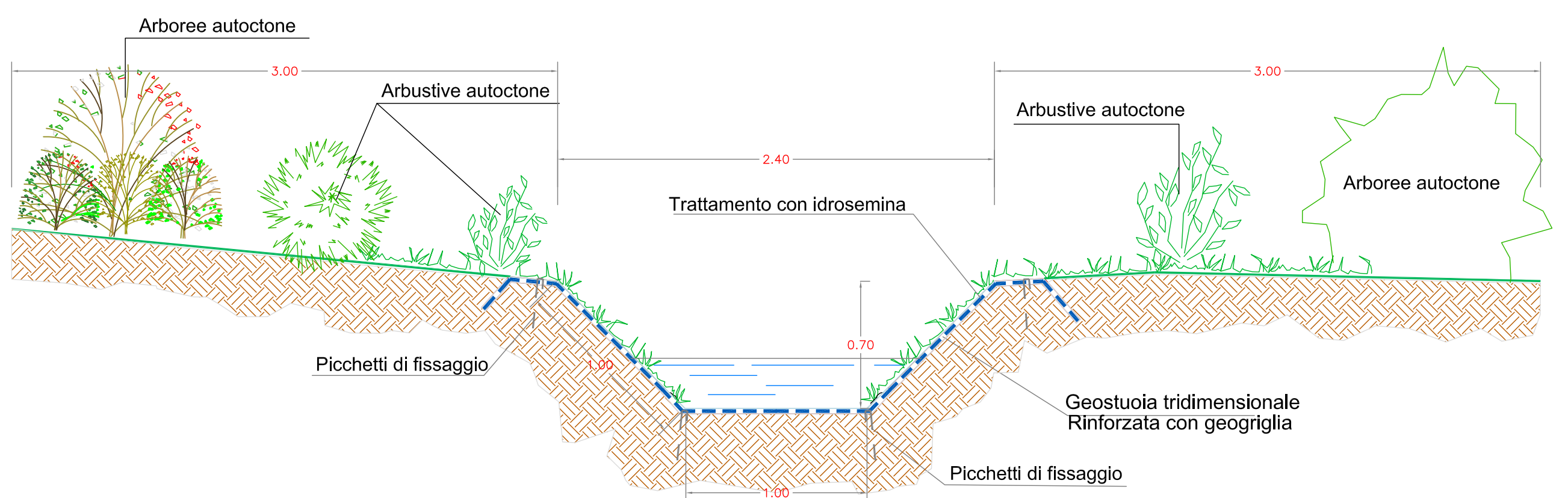
Particolare di massima - Sezione tipo Fosso Casalta Scala 1:50
