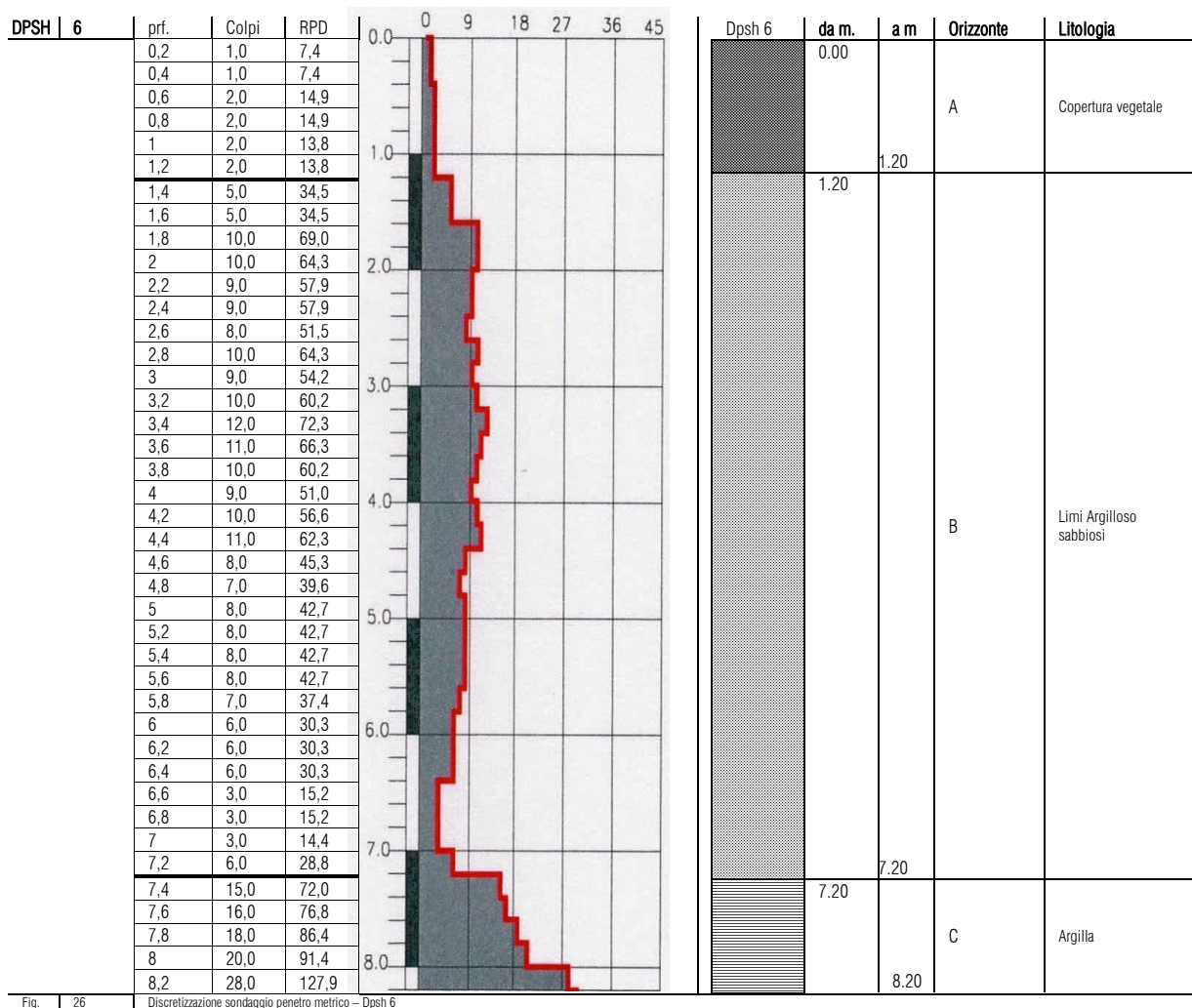
Fig. | 26 | Discretizzazione sondaggio penetrometrico - Dpsh 6
