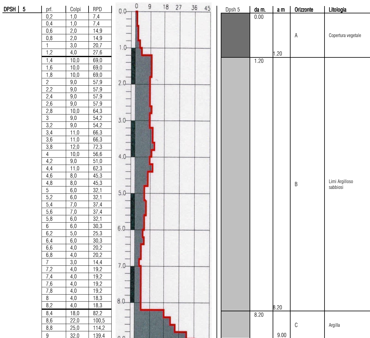
Fig. | 25 | Discretizzazione sondaggio penetrometrico – Dpsh 5
