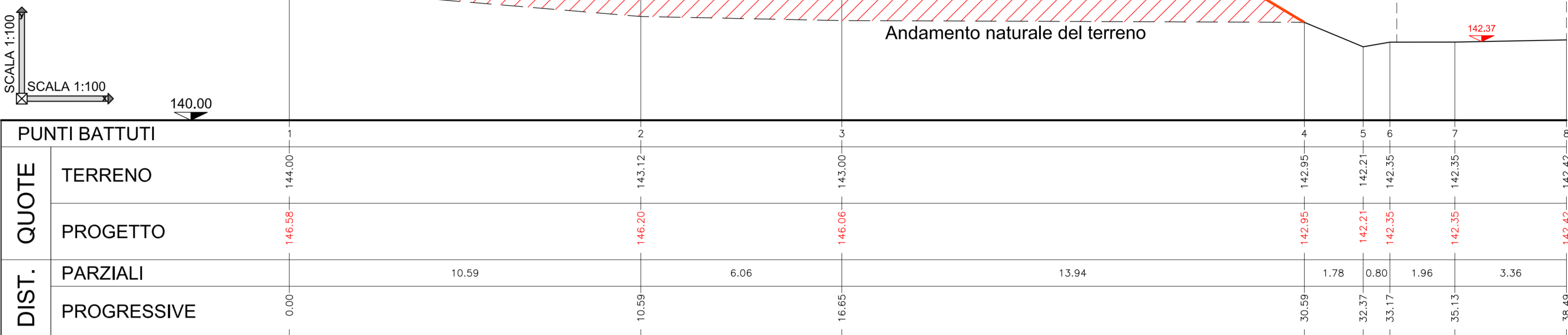
PROFILO 7-7
